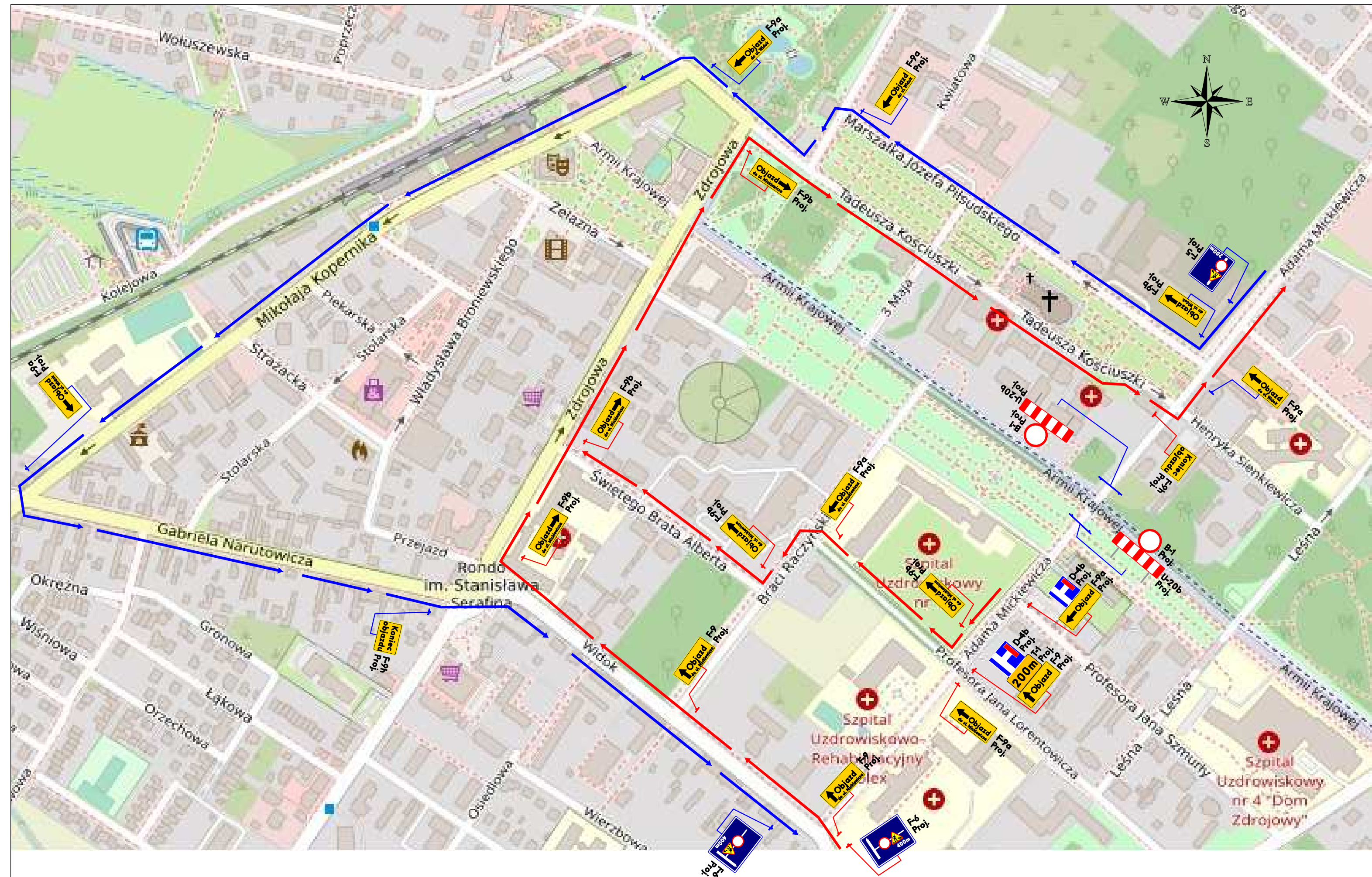
Oznakowanie objazdów na czas realizacji zadania "Przebudowa deptaka przy alei Armii Krajowej w Ciechocinku"
